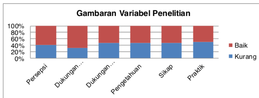
Gambar 1. Grafik Distribusi Frekuensi Variabel Penelitian
