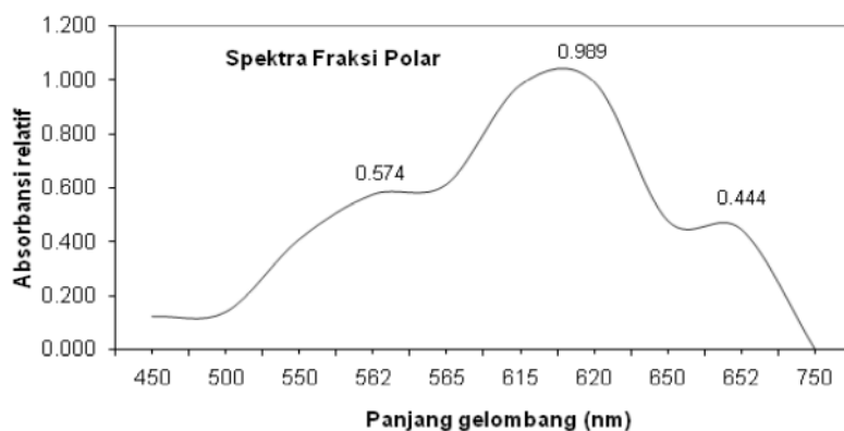
Gambar 1. Spektra ekstrak pigmen polar (dalam buffer NaOH-KH 2 PO 4 (pH 7) dari Spirulina sp. kering (pengenceran 10x)
