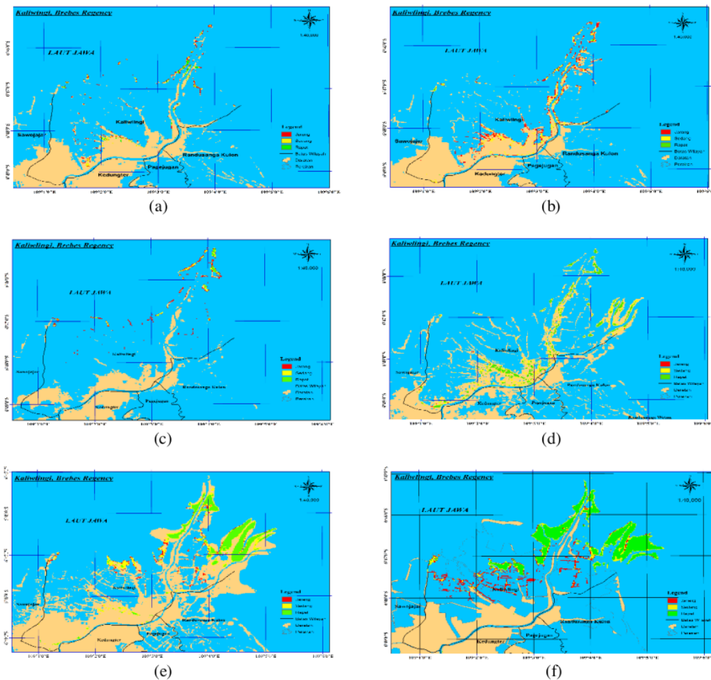
Gambar 1. Peta Sebaran Ekosistem Mangrove di Desa Kaliwlingi, Kabupaten Brebes a) Tahun 1996; b) Tahun 2000; c) Tahun 2007; d) Tahun 2010; e) Tahun 2015; f) Tahun 2019.
