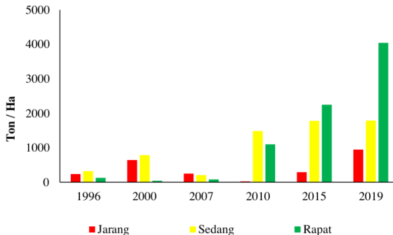
Gambar 3. Grafik Prediksi Simpanan Karbon Tahun 1996 - 2019 pada Kerapatan Jarang, Sedang, Rapat di Desa Kaliwlingi, Kabupaten Brebes.
