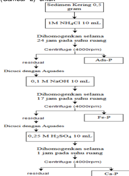
Gambar 2. Diagram alir penentuan fraksi fosfat (SEDEX).
