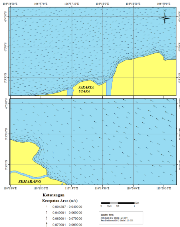
Gambar 3. Pola arus kondisi surut menuju pasang.
