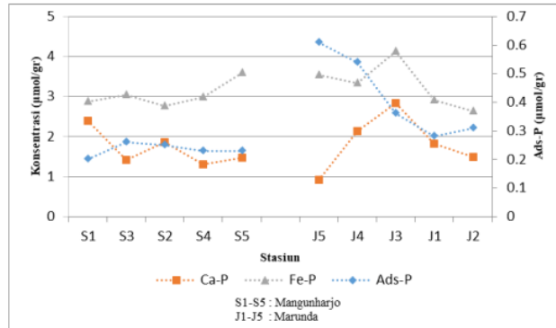
Gambar 4. Grafik fluktuasi konsentrasi fraksi fosfat dalam sedimen
