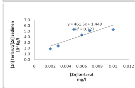
Gambar 4. Model Partisi Logam Pb, Cu dan Zn pada sistem fase terlarut terhadap partikel dalam air
