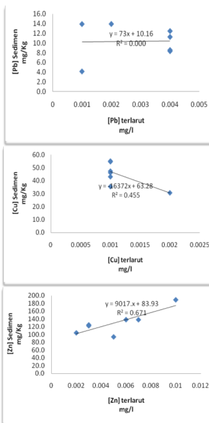
Gambar 1. Model Partisi Logam Pb, Cu dan Zn pada sistem fase terlarut terhadap sedimen
