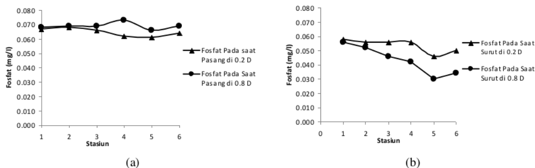
Gambar 3. Konsentrasi fosfat ( \text{PO}_4^{3-} ) pada saat pasang (a) dan pada saat surut (b) di Muara Sungai Demaan Jepara
