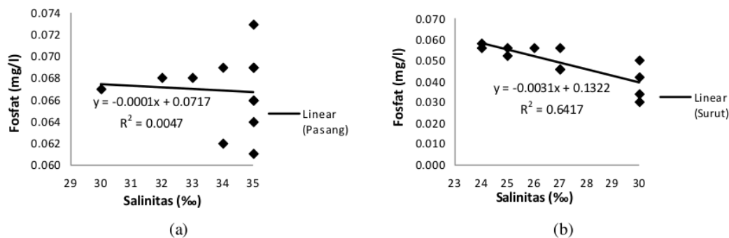
Gambar 4. Hubungan konsentrasi fosfat terhadap salinitas pada kondisi (a) Pasang dan (b) Surut
