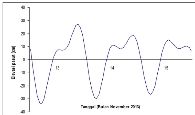
Gambar 2. Hasil peramalan pasang surut dengan software Naotide
