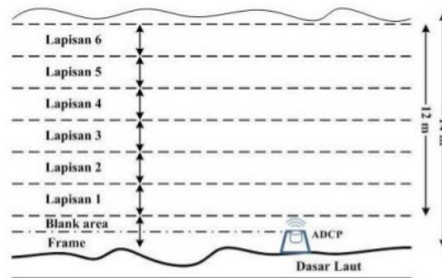
Gambar 2. Ilustrasi lapisan kedalaman pengukuran
