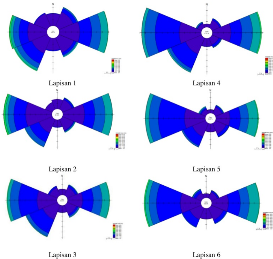
Gambar 4. Current Rose untuk tiap lapisan kedalaman pengukuran
