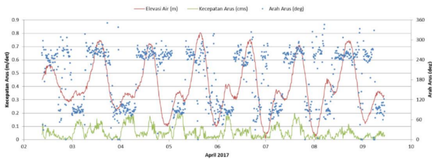
Gambar 5. Grafik karakteristik arus
