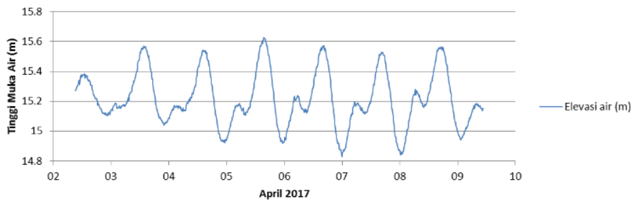
Gambar 3. Elevasi muka air Perairan Pulau Cilik, Karimunjawa
