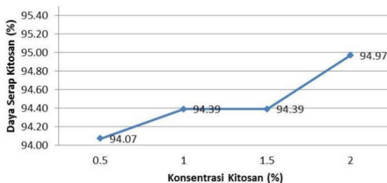
Gambar 2. Daya Serap Kitosan terhadap Logam Berat Pb
