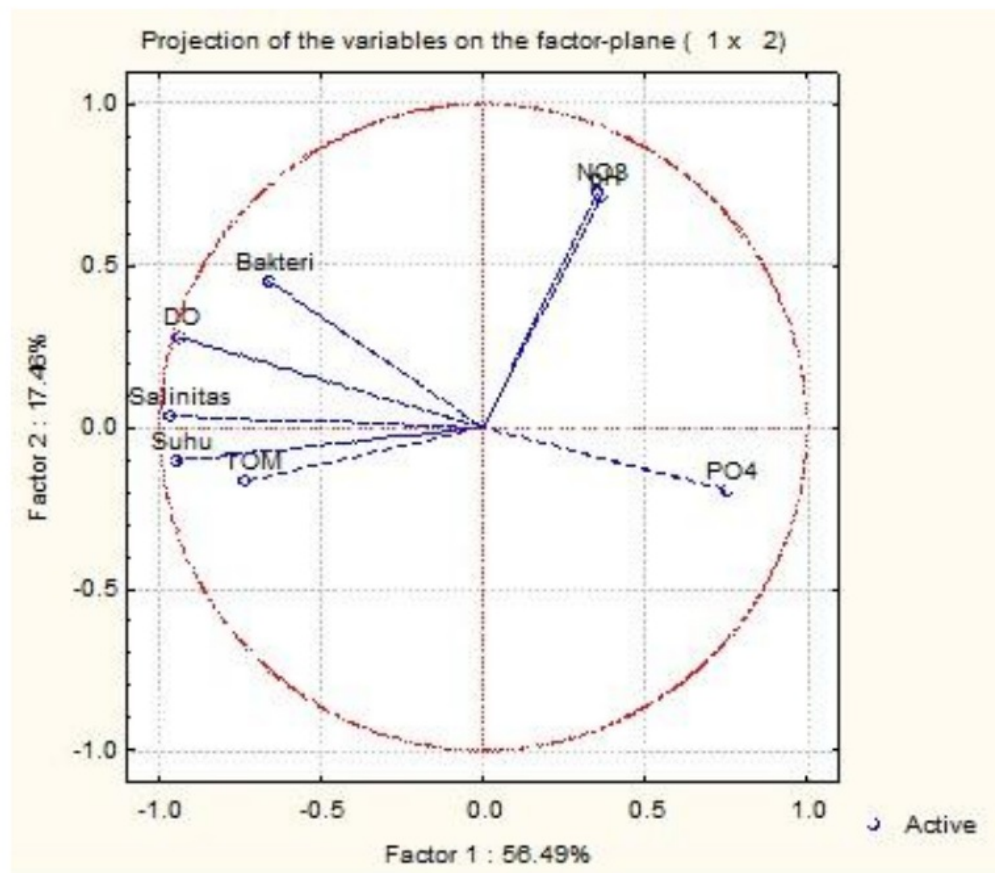
Gambar 3. Grafik PCA (Principal Component Analysis).
