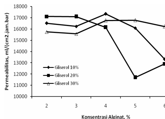
Gambar 2. Pengaruh konsentrasi alginat terhadap permeabilitas film
