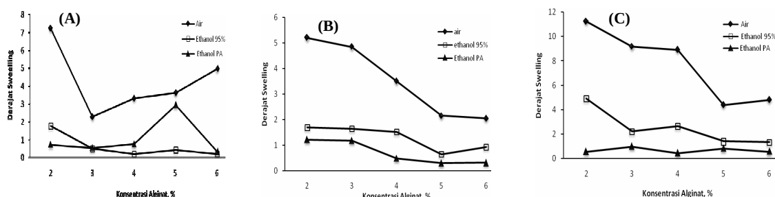
Gambar 4. Pengaruh konsentrasi alginat terhadap derajat swelling dengan penambahan gliserol: (A) 10%, (B) 20%, dan C) 30%
