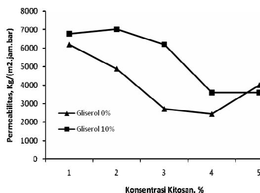
Gambar 1. Pengaruh konsentrasi kitosan terhadap permeabilitas film
