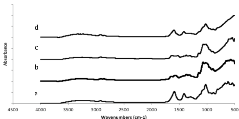
Gambar 5. Hasil uji FTIR dari film : a. alginat (AG); b. kitosan; c. AG-CH; d. AG/CH
