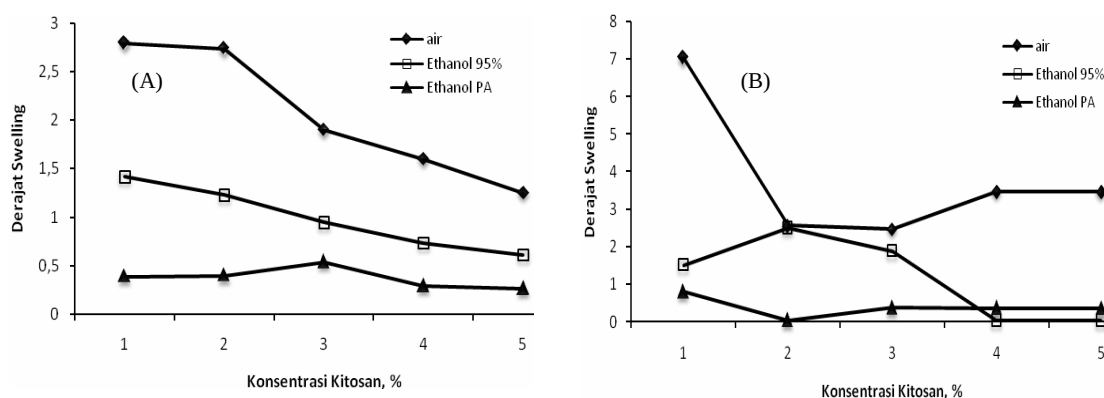
Gambar 3. Pengaruh konsentrasi kitosan terhadap derajat swelling: (A) tanpa penambahan gliserol, (B) dengan penambahan 10% gliserol
