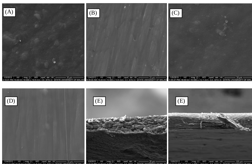
Gambar 6 : Hasil Uji SEM: (A) permukaan AG; (B) permukaan CH; (C) permukaan AG/CH; (D) permukaan AG-CH; (E) penampang AG/CH; (F) penampang AG-CH.
