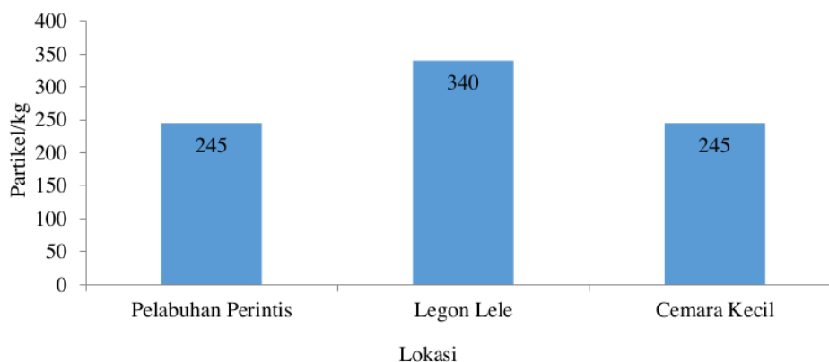
Gambar 3. Kelimpahan Mikroplastik pada Sedimen Berdasarkan Lokasi
