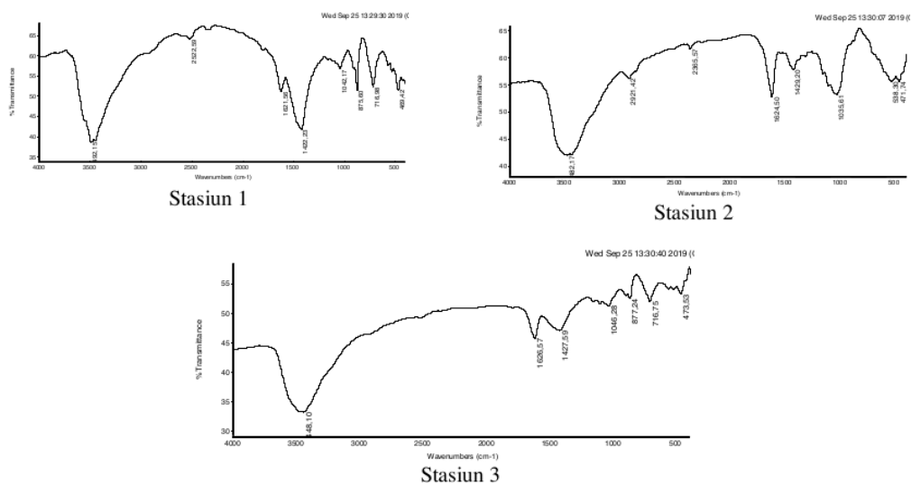
Gambar 5. Spektrum IR Mikroplastik Lokasi Pelabuhan Perintis
