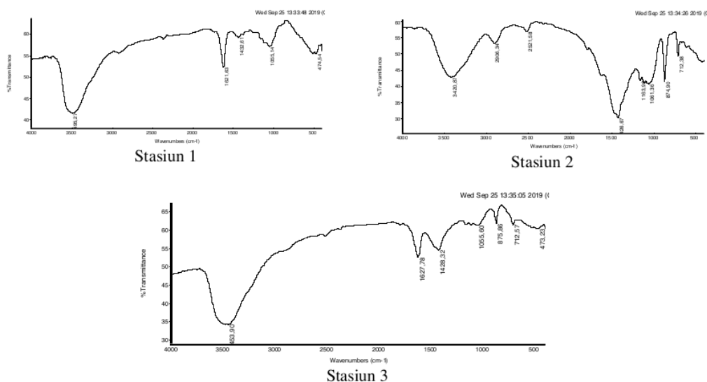
Gambar 6. Spektrum IR Mikroplastik Lokasi Legon Lele
