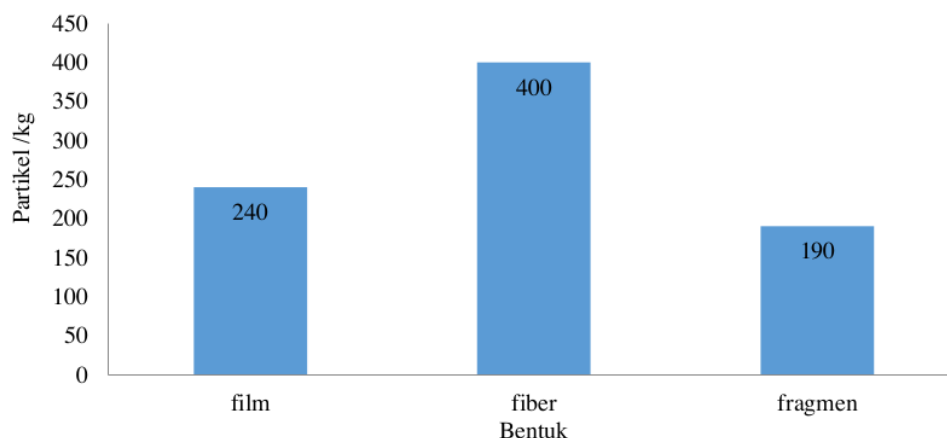
Gambar 4. Kelimpahan Mikroplastik pada Sedimen Berdasarkan Bentuk
