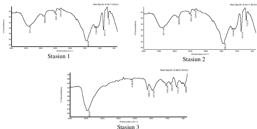
Gambar 7. Spektrum IR Mikroplastik Lokasi Cemara Kecil
