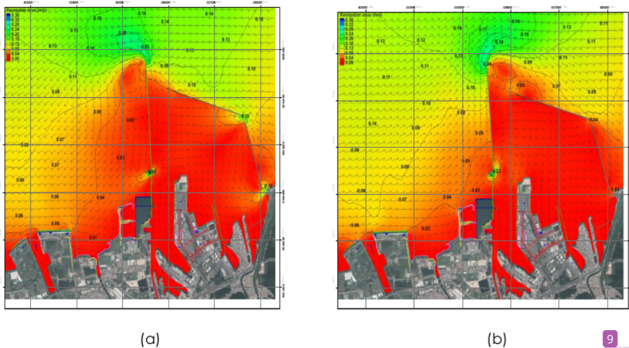
Gambar 4. Model Kecepatan dan Arah Arus Pada Kondisi Setelah Reklamasi, (a) surut menuju pasang, (b) pasang menuju surut.
