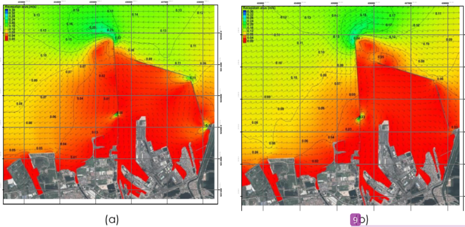
Gambar 3. Model kecepatan dan arah arus pada kondisi eksisting, (a) surut menuju pasang, (b) pasang menuju surut.
