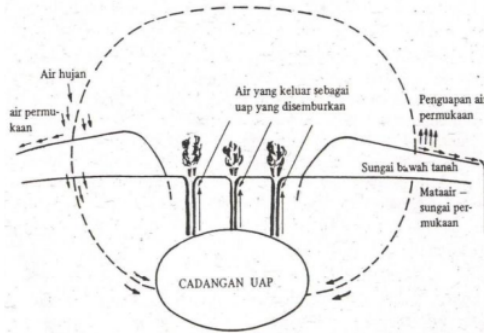
Gambar 3. Daur Hidrologi Panas Bumi [1]
