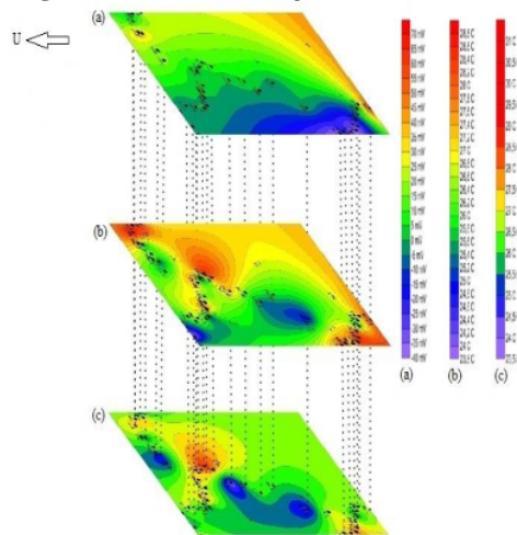
Gambar 11. Overlay peta kontur sebaran SP terhadap peta kontur sebaran suhu permukaan dangkal, (a) kontur sebaran SP, (b) kontur sebaran suhu permukaan dangkal kedalaman 50cm dan 100cm.
