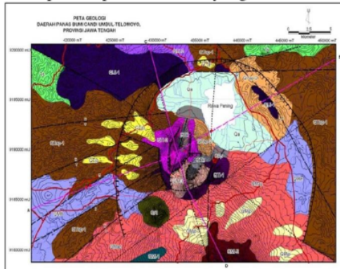
Gambar 1. Peta geologi daerah panas bumi Candi Umbul-Telomoyo [18]
