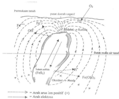
Gambar 4. Mekanisme polarisasi pada tubuh mineral [15]
