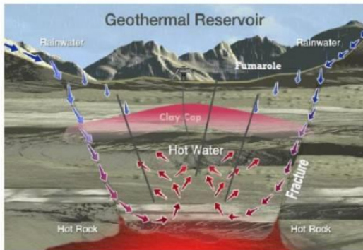
Gambar 2. Sistem Panas Bumi [4]
