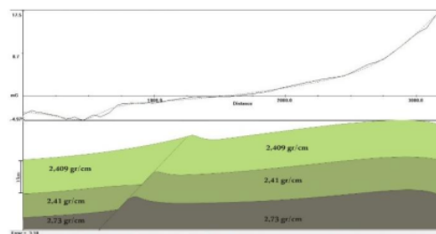
Gambar 7 Pemodelan 2D Data Gravitasi pada Sayatan B
