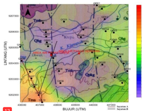
Gambar 5 Kontur Anomali Bouguer Lengkap di Topografi Daerah Penelitian
