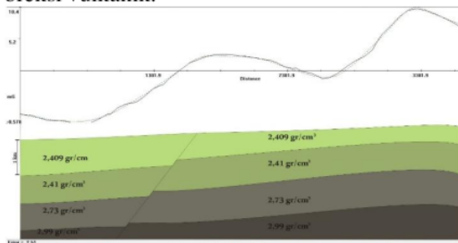
Gambar 6 Pemodelan 2D Data Gravitasi pada Sayatan A
