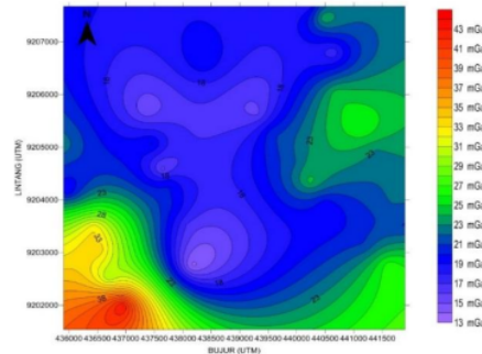
Gambar 4 Kontur Anomali Bouguer Lengkap
