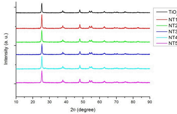
Figure 1. XRD analyses of TiO 2 and N-doped TiO 2 .
