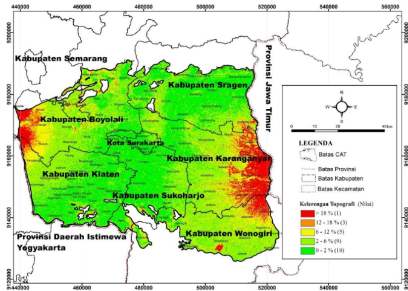
Gambar 8. Peta Topografi
