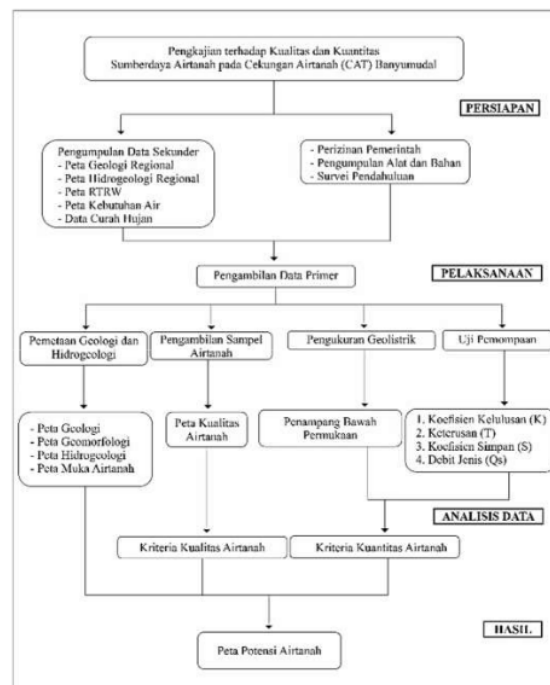
Gambar 4. Metodologi Penelitian
