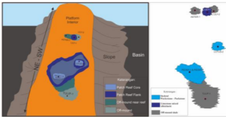
Gambar 5. Persebaran Fasies Formasi Tuban (Miosen Awal)
