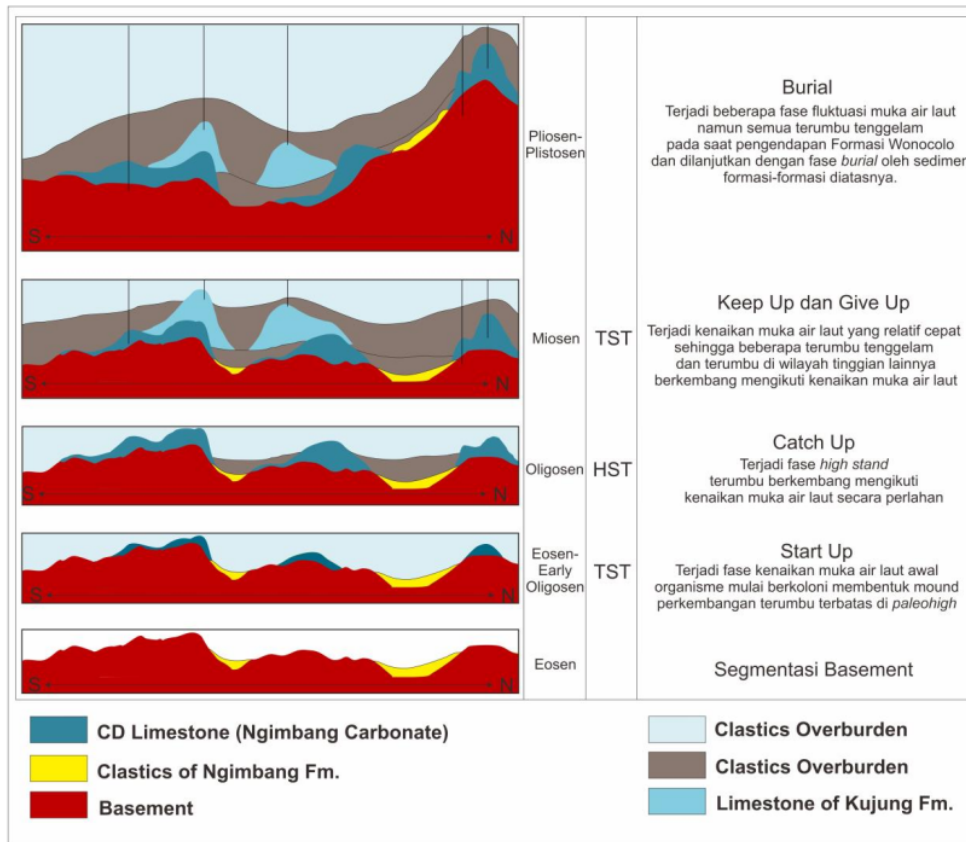
Gambar 6. Perkembangan Terumbu Formasi Kujung dan Tuban
