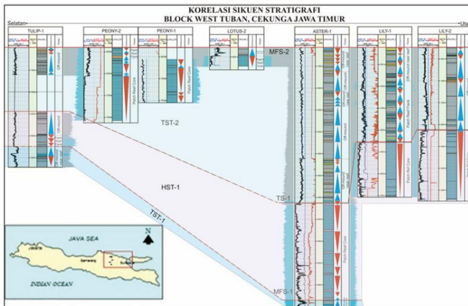
Gambar 3. Sikuen Stratigrafi Formasi Kujung dan Tuban.
