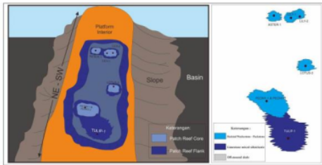
Gambar 4. Persebaran Fasies Formasi Kujung (Oligosen – Miosen).
