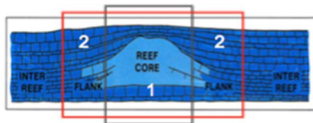
Gambar 1. Fasies Pengendapan pada Patch reef (James, 1979). Kotak abu-abu (nomor 1) adalah fasies Core-patch reef . Kotak merah (nomor 2) adalah fasies flank-patch reef .
