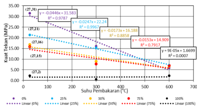
Gambar 5. Hubungan antara Kuat Tekan dengan Suhu Pembakaran Beton Pumice
