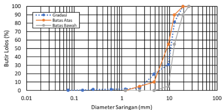
Gambar 3. Grafik analisa saringan batu pumice
