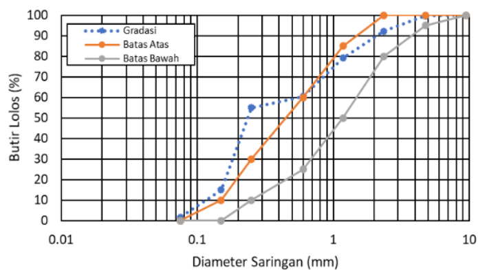
Gambar 2 Grafik analisa saringan Pasir Muntitan
