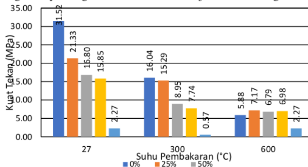
Gambar 4. Perbandingan kuat tekan beton
