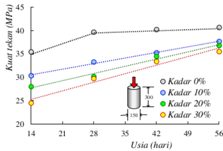
Gambar 8. Respon perkembangan kuat tekan sebagai fungsi waktu
