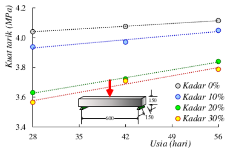
Gambar 10. Respon perkembangan kuat tarik sebagai fungsi waktu
