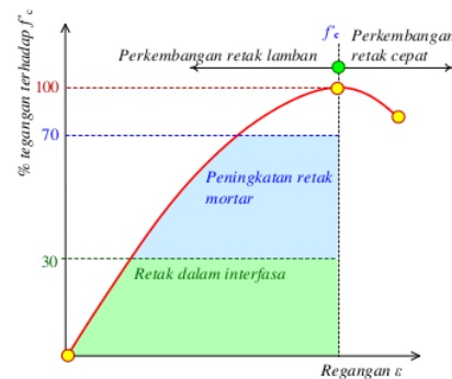
Gambar 3. Pola keruntuhan material beton
