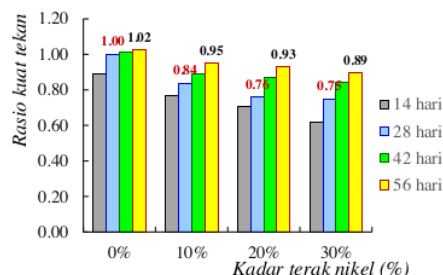
Gambar 5. Respon kuat tekan beton terak nikel
