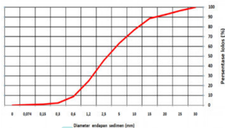
Gambar 6. Gradasi material endapan dasar sungai di Check Dam Linggasari 27 Mei 2009 (Soewarno & Sukatja, 2010)
