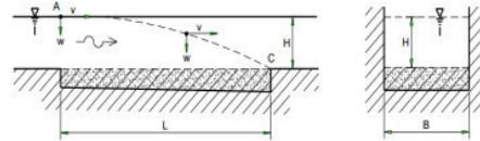
Gambar 1. Sketsa kantong lumpur (Kementerian Pekerjaan Umum, 2013)
