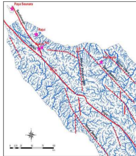
Gambar 4. Pola Aliran Sungai di Provinsi NAD
