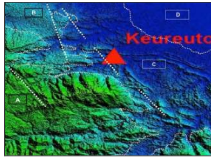
Gambar 7. Kondisi Morfotektonik Disekitar Bendungan Keureuto Provinsi NAD
