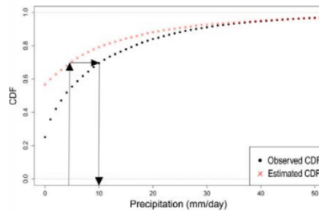
Gambar 1. Skema metode quantile mapping
