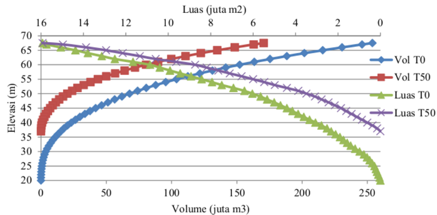
Gambar 4. Lengkung Kapasitas-Luas tampungan Waduk Karian
