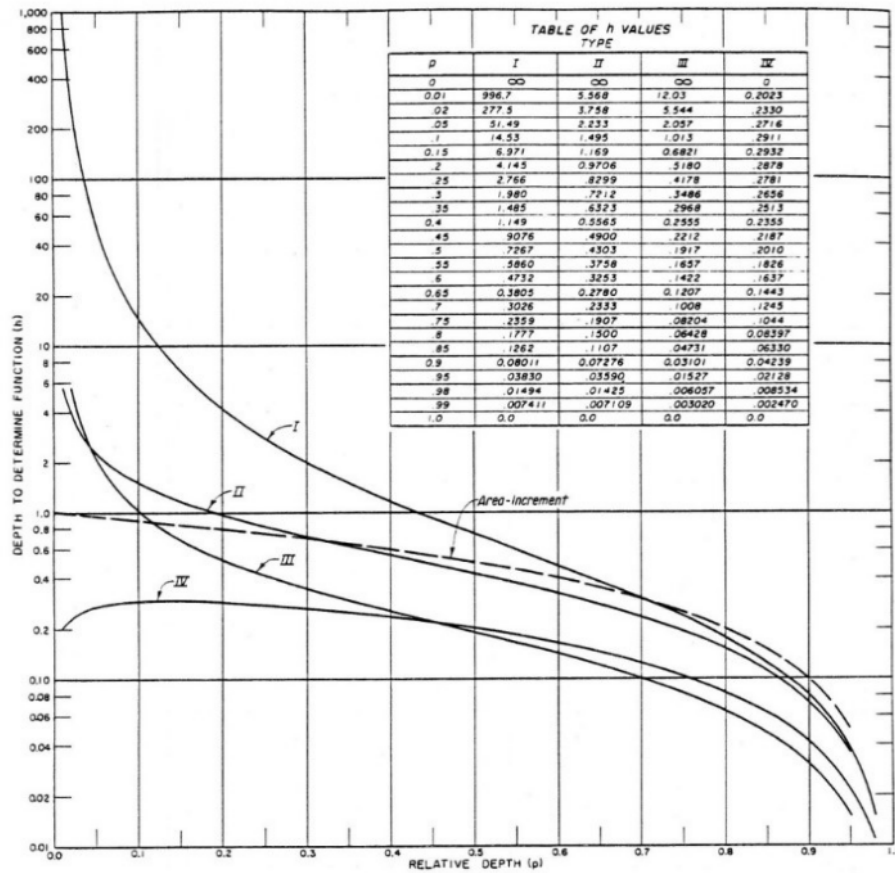
Gambar 2. Hubungan Kedalaman Relatif dan Nilai F (Morris & Fan, 2009)
