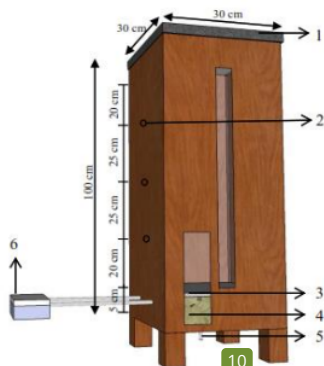
Gambar 1. Skema reaktor biodrying , (1) penutup reaktor, (2) lubang pengukuran suhu, (3) kawat jarring, (4) susunan kerikil, (5) saluran lindi, (6) aerator
