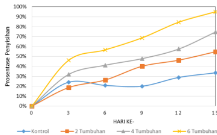
Gambar 3. Grafik efisiensi penyisihan kromium (Cr) total selama operasional reaktor
