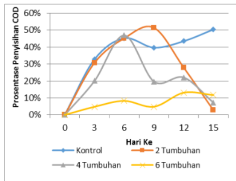
Gambar 5. Grafik efisiensi penyisihan COD selama operasional reaktor
