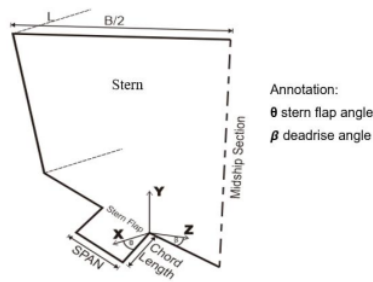
Figure 2. Stern flap parameter
