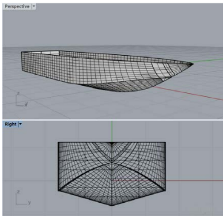
Gambar 4. Kapal Patroli Tanpa Bilge Keel
