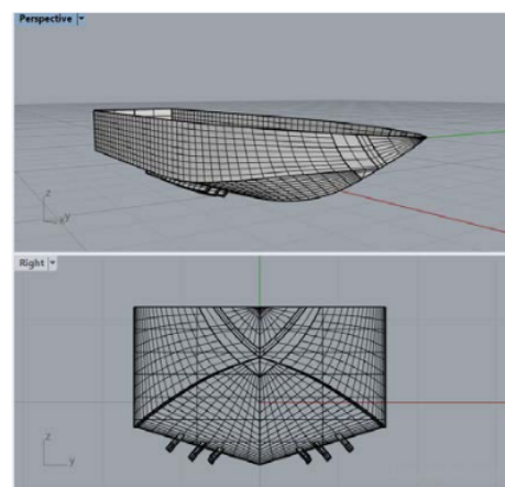
Gambar 7. Kapal Patroli dengan Bilge Keel 3 Pasang
