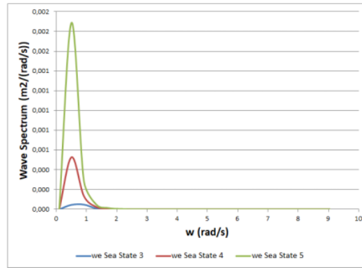
Gambar 8. Spektrum Gelombang
