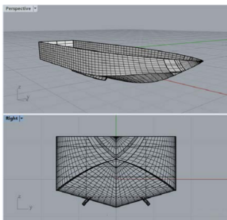
Gambar 5. Kapal Patroli dengan Bilge Keel 1 Pasang
