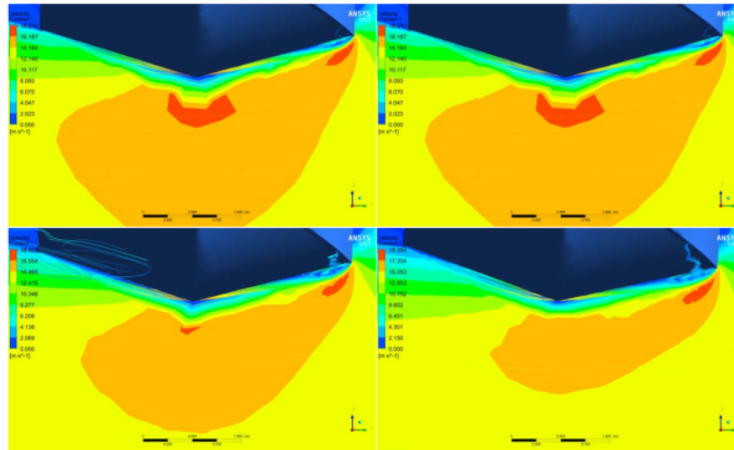
Gambar 15. Kontur Kecepatan Rolling Kapal Model Tanpa Bilge Keel
