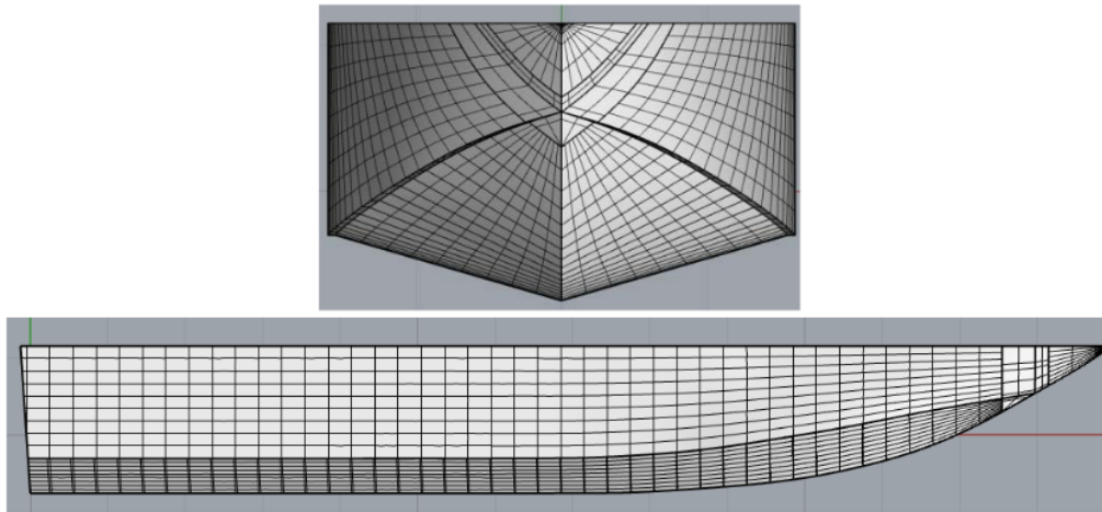
Gambar 1. Desain Geometri 3-D Kapal Patroli
