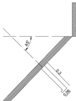
Gambar 3. Desain Bilge Keel
