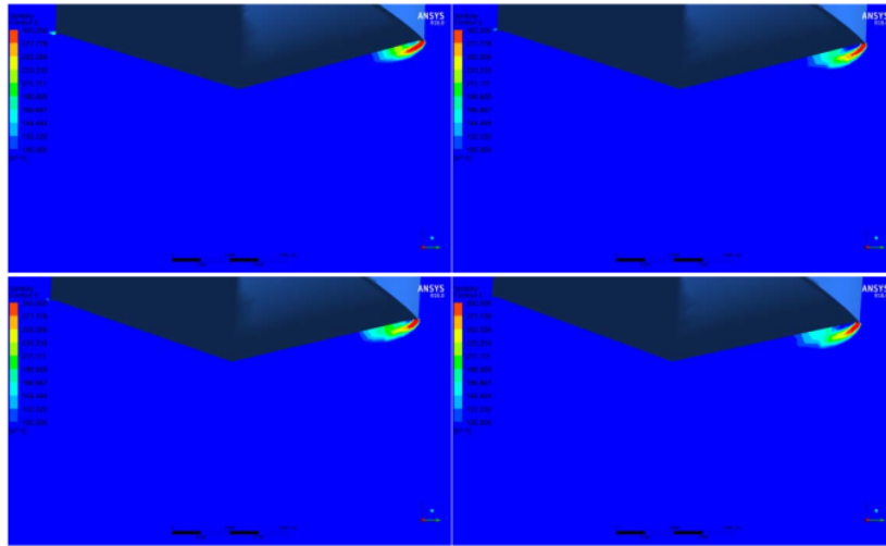
Gambar 13. Vorticity Kapal Tanpa Bilge Keel
