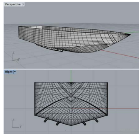
Gambar 6. Kapal Patroli dengan Bilge Keel 2 Pasang
