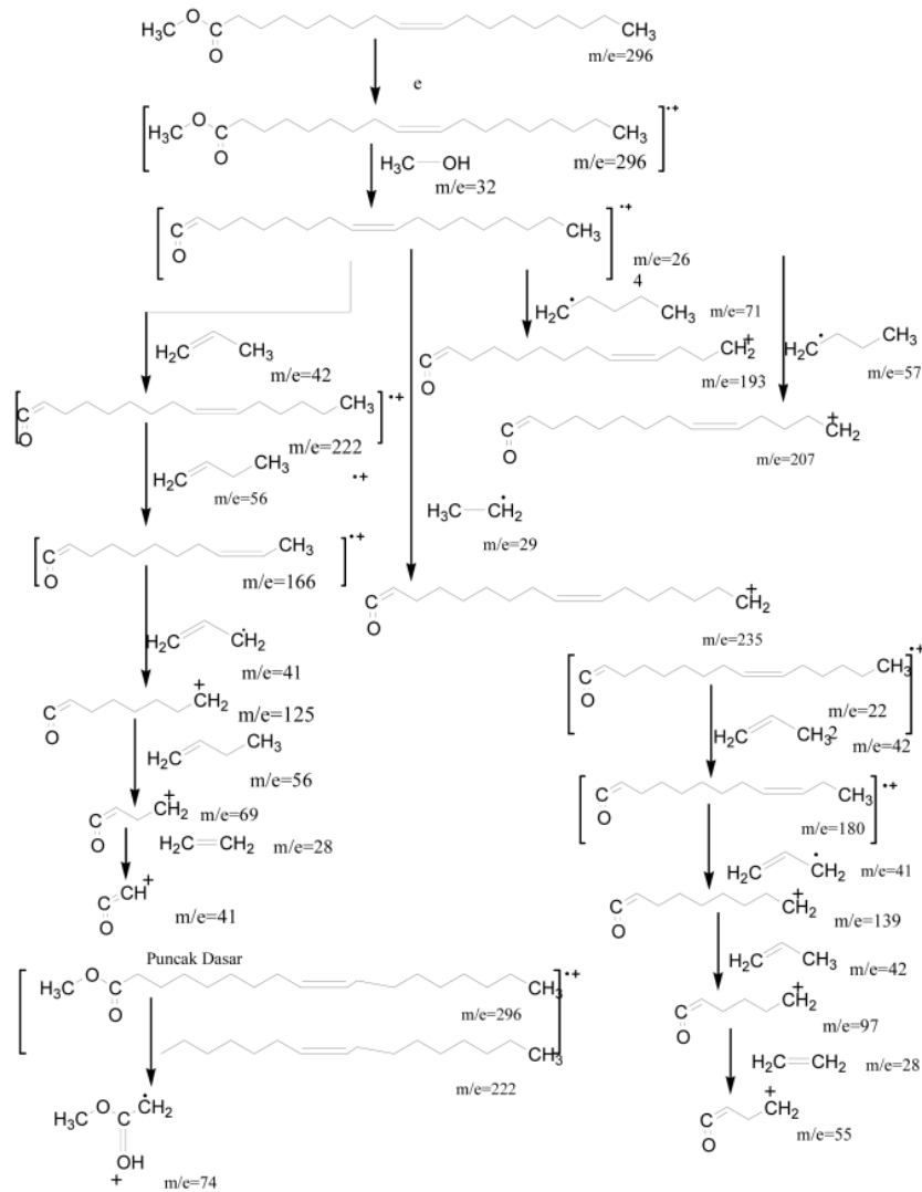
Gambar 2. Skema puncak-puncak dari spectrum
