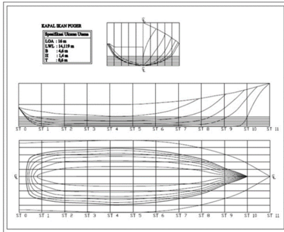
Gambar 4. Linesplan lambung kapal ikan puger.
