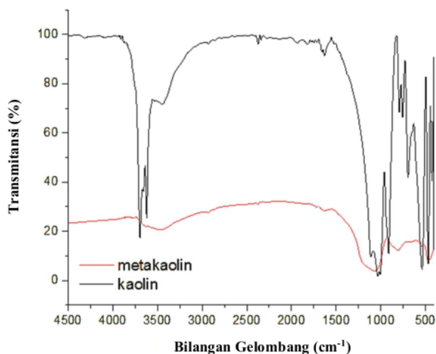
Gambar 3. Hasil analisis FTIR kaolin dan metakaolin.
