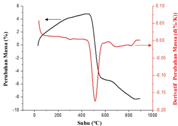
Gambar 1. Hasil analisis termogravimetri kaolin.
