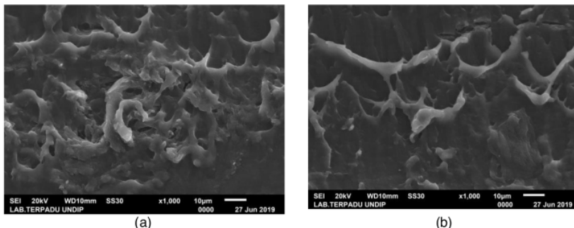
Gambar 8. Mikrograf SEM bioplastik dengan pemlastis gliserol (a) dan sorbitol (b)
