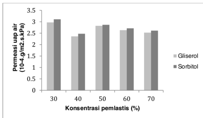
Gambar 4. Permeasi uap air bioplastik dengan pemlastis gliserol dan sorbitol pada berbagai konsentrasi
