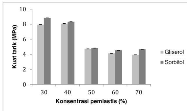
Gambar 1. Kuat tarik bioplastik dengan pemlastis gliserol dan sorbitol pada berbagai konsentrasi
