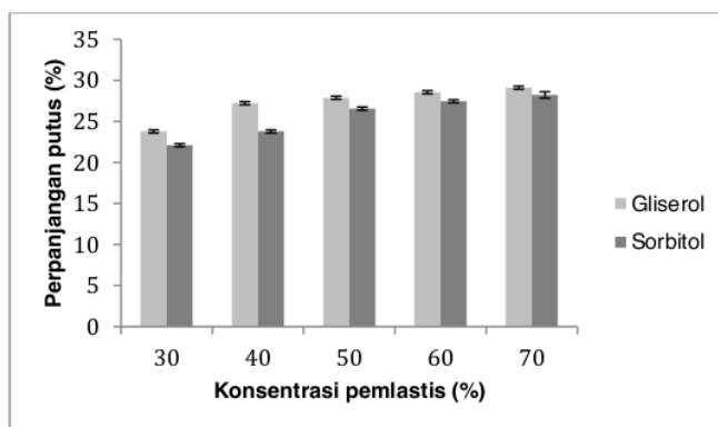
Gambar 2. Perpanjangan putus bioplastik dengan pemlastis gliserol dan sorbitol pada berbagai konsentrasi
