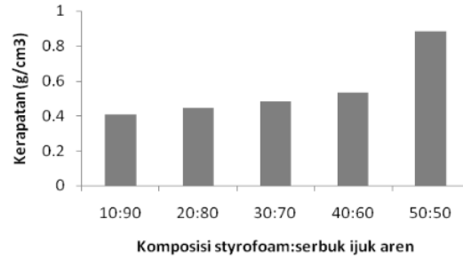
Gambar 3. Kerapatan komposit pada berbagai komposisi styrofoam dan serbuk ijuk aren.
