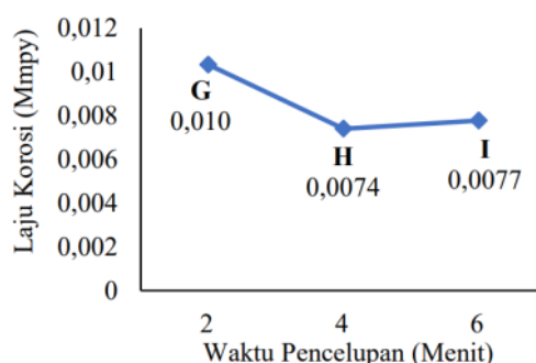
Gambar 6. Laju korosi pada temperatur 480°C
