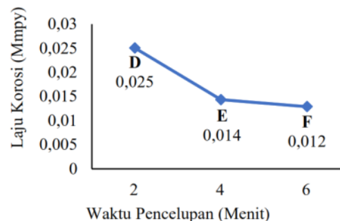
Gambar 5. Laju korosi pada temperatur 455°C
