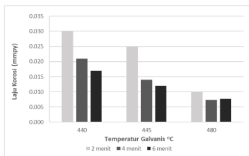
Gambar 7. Perbandingan korosi berdasarkan waktu dan temperatur
