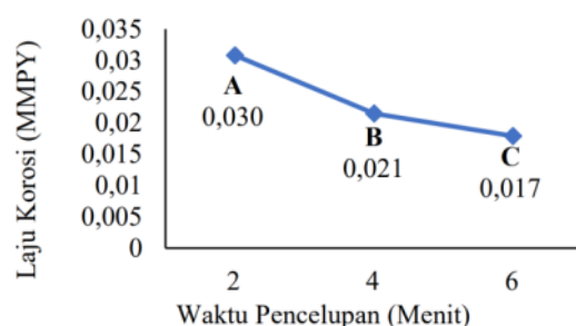
Gambar 4. Laju korosi pada temperatur 440°C
