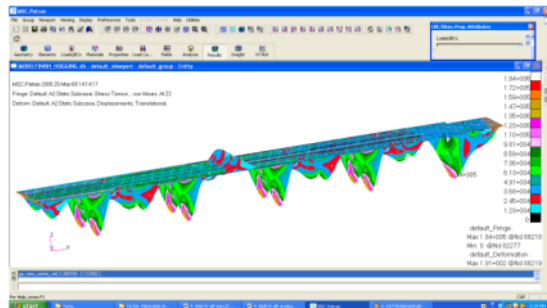
Kondisi Hogging
