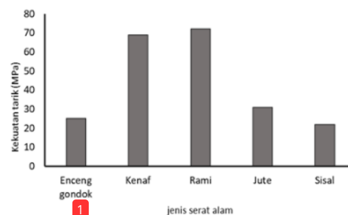
Gambar 5. Kekuatan Tarik Komposit Poliester dengan Penguat Serat Alam (Simonassi, dkk., 2017; Prasad, dkk., 2009; Hanamanagouda, dkk., 2016; Abiral, dkk., 2014).
