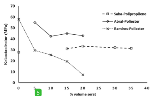
Gambar 3. Pengaruh fraksi volume terhadap kekuatan lentur komposit dengan penguat serat enceng gondok (Saha, 2011; Abiral dkk., 2013; Ramirez dkk., 2015)
