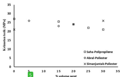
Gambar 2. Pengaruh fraksi volume terhadap kekuatan tarik komposit dengan penguat serat enceng gondok (Saha, 2011; Simanjuntak, 2013; Abiral dkk., 2014)
