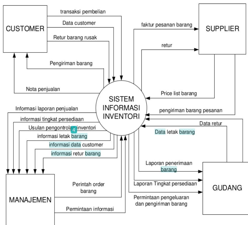
Gambar 4 Context diagram sistem informasi
