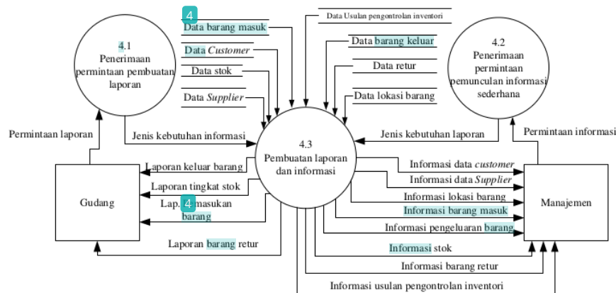
Gambar 11 DFD level 1 pembuatan laporan dan informasi
