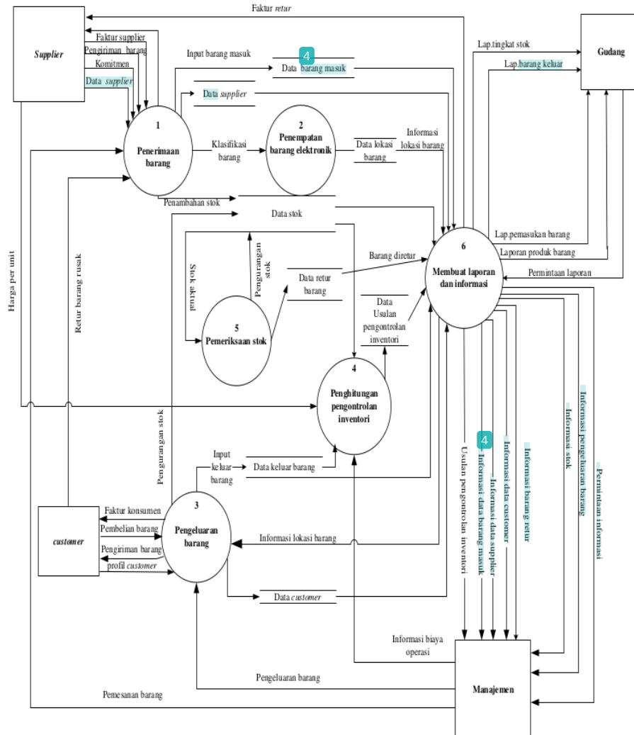
Gambar 5 DFD level 0 sistem informasi
