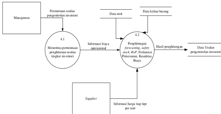
Gambar 9 DFD level 1 penghitungan pengontrolan inventori
