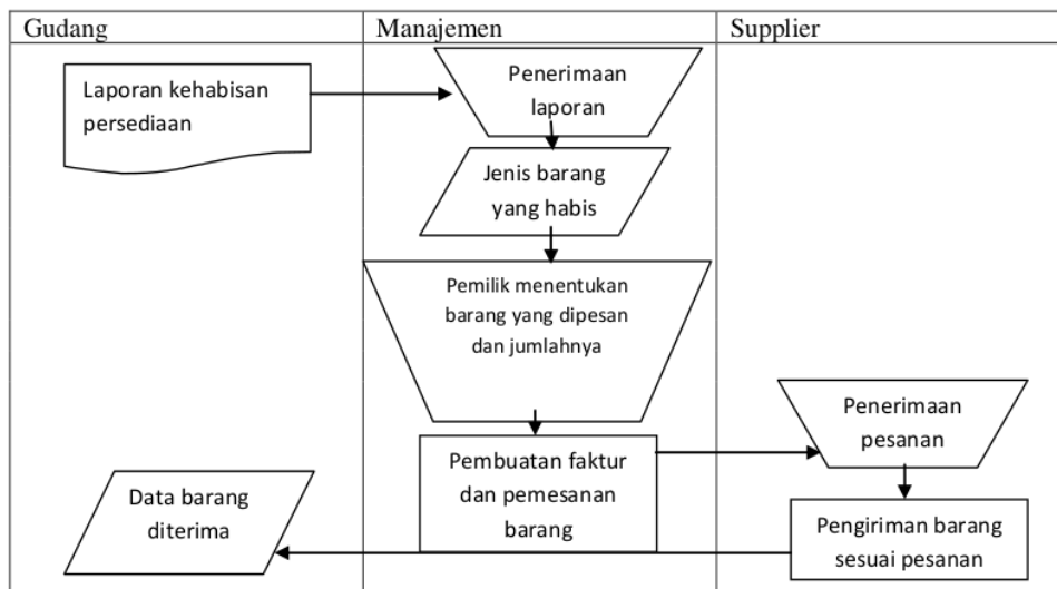
Gambar 3 Prosedur pengontrolan persediaan saat ini
