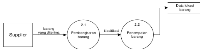
Gambar 7 DFD level 1 penempatan barang
