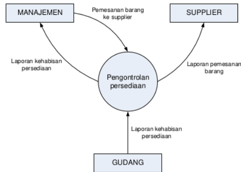
Gambar 2 Context diagram sistem saat ini
