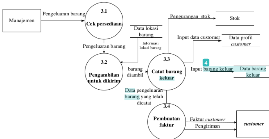
Gambar 8 DFD level 1 pengeluaran barang
