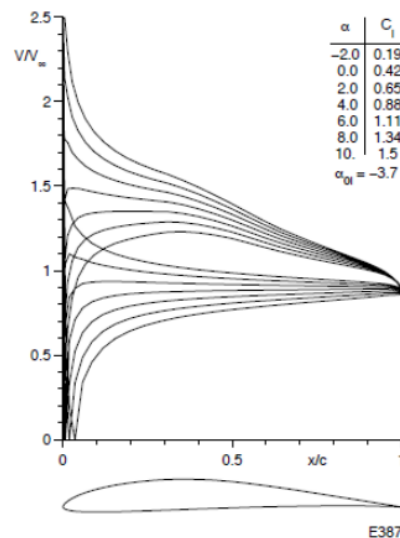
Gambar 7. Distribusi kecepatan tangensial dan profil airfoil E387
