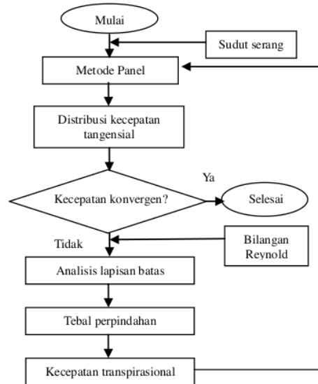
Gambar 1. Diagram alir metoda interaksi viskos – tak viskos
