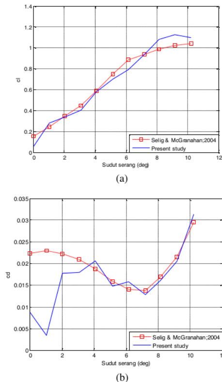
Gambar 12. 10 Koefisien gaya angkat dan (b) koefisien gaya hambat airfoil S822 untuk Re = 200000
