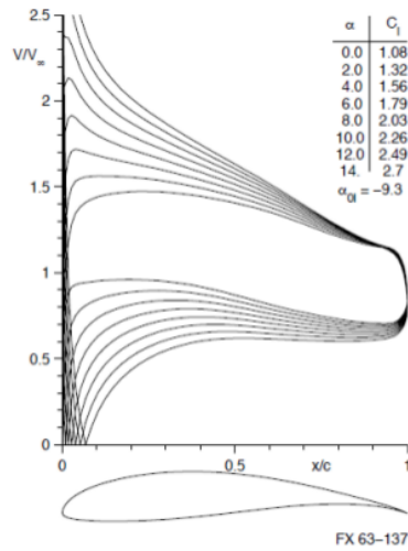
Gambar 9. Distribusi kecepatan tangensial dan profil airfoil FX 63-137
