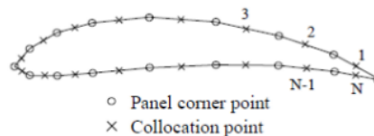
Gambar 3. Pembuatan panel pada airfoil
