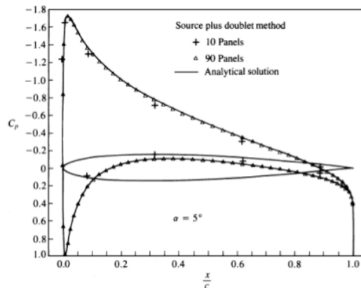
Gambar 4. Distribusi tekanan airfoil simetri dengan 10 dan 90 panel [6].
