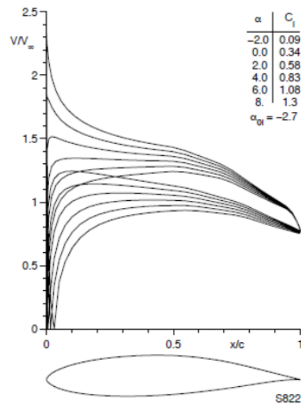
Gambar 11. Distribusi kecepatan tangensial dan profil airfoil S822
