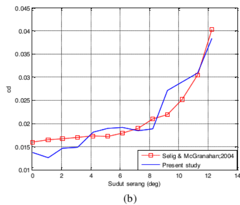
Gambar 10. Koefisien gaya angkat dan (b) koefisien gaya hambat airfoil FX 63-137 untuk Re = 200000
