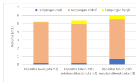
Gambar 6. Perubahan kapasitas tampungan Waduk Gunungrowo pada tiap fungsi tampungan
