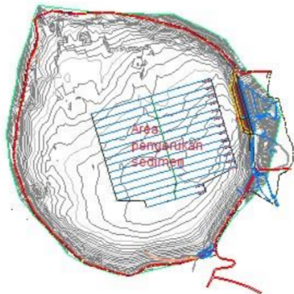
Gambar 5. Peta bathimetri Waduk Gunungrowo tahun 2015 [18]
