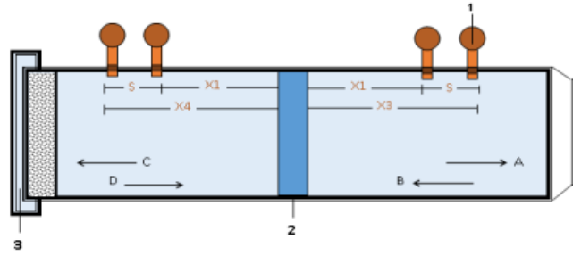
Gambar 4.3. Tabung impedansi memiliki 4 mikrofon pada uji Sound Transmission Loss [28]
