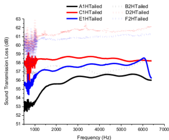
Gambar 4.6. Perbandingan uji STL BiomassaFRP dengan rongga berekor tunggal-multipel[28]
