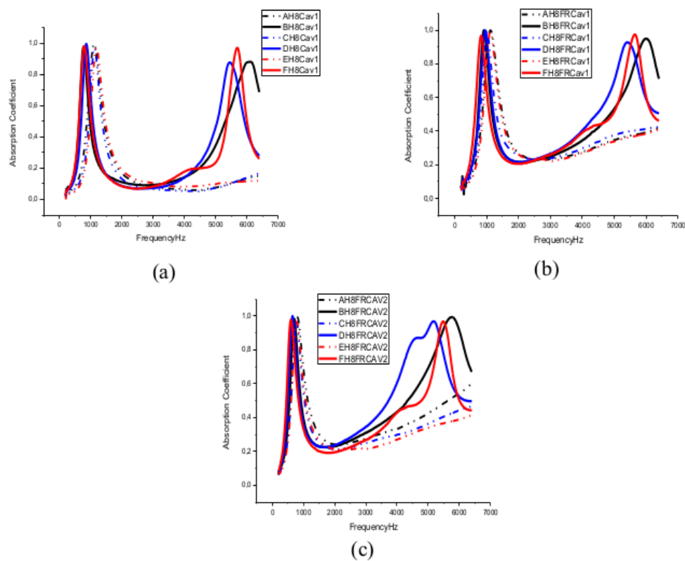
Gambar 3.8. (a) Koefisien penyerapan cangkang komposit : rongga 10 mm, (b) lapisan berserat dan rongga 10 mm, (c) lapisan berserat dan rongga 20 mm[13]
