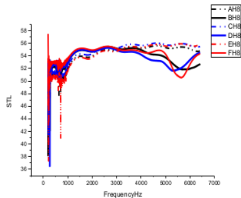
Gambar 3.10. STL SFRP dengan 8 lubang resonator[13]
