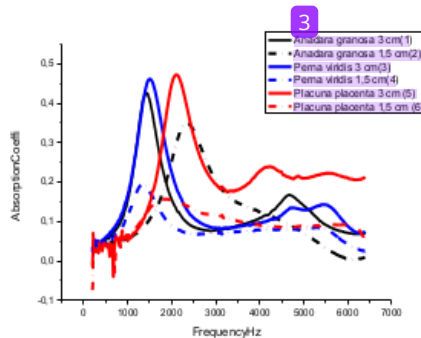
Gambar 3.4. Koefisien penyerapan komposit kerang tanpa perlakuan[13]
