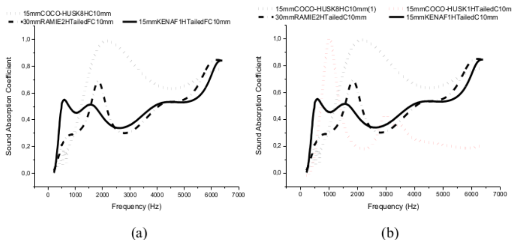
Gambar 4.9. Perbandingan Penyerapan serat sabut kelapa dalam penelitian sebelumnya dan Bahan biomassa dengan rongga berekor[28]
