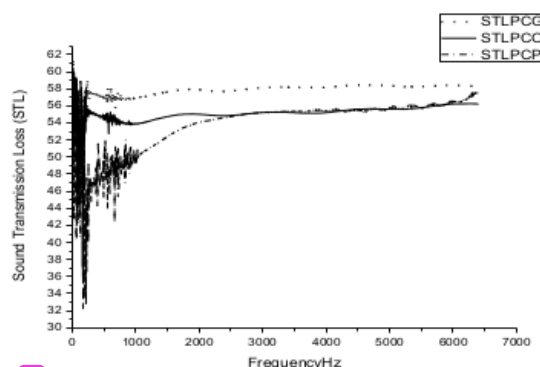
Gambar 2.14. Sound Transmission Loss (STL) dari PCG, PCO dan PCP
