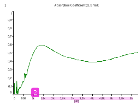
Gambar 2.3. Grafik Koefisien Absorpsi mortar cangkang kerang tebal 0,8 cm
