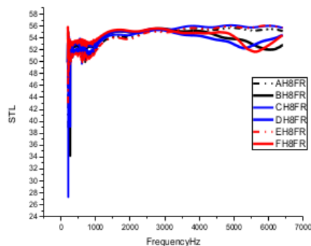
Gambar 3.11. STL SFRP dengan kombinasi resonator dan lapisan serat[13]
