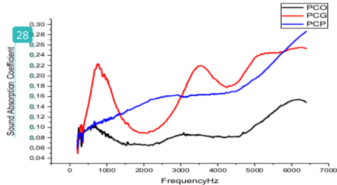
Gambar 2.10. Hasil Uji Koefisien Absorpsi
