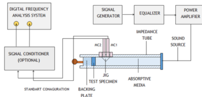
Gambar 4.2. Pengukuran Koefisien Serapan menggunakan tabung impedansi B&K mengacu pada ASTM E 1050-98 [28,29]
