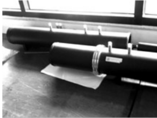
14 Gambar 2.12. Tabung Impedansi dengan mikrofon
