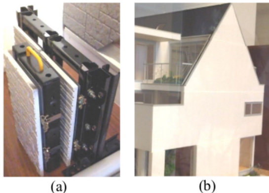
Gambar 5.5. (a) Rencana panel dinding lapis ganda dengan komposit serat alam (FRP) sebagai lapis kedua, (b) konsep modern rumah terang dengan panel dinding ganda yang terang [12]
