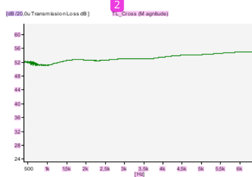
Gambar 2.6. STL mortar cangkang kerang tebal 1.8 cm
