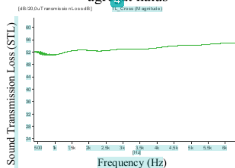
Gambar 5.3. Sound Transmission Loss beton foamed dengan cangkang kerang ebagai agregat halus
