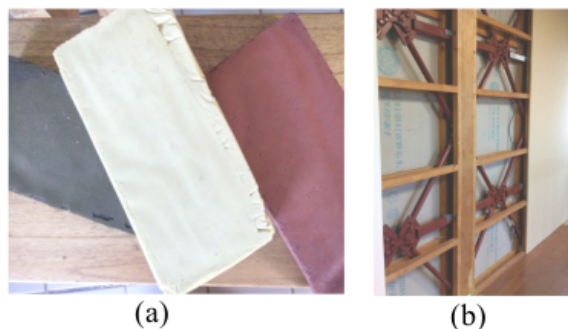
Gambar 5.4. (a) Beton Foamed dengan cangkang kerang sebagai agregat halus untuk panel dinding (b) Konsep panel lapis ganda pada dinding
