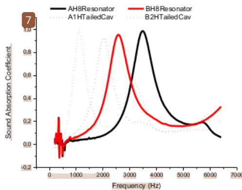
Gambar 4.8. Perbandingan Penyerapan poliester yang diperkuat serat sekam kelapa antara penelitian sebelumnya dan penelitian ini[28]
