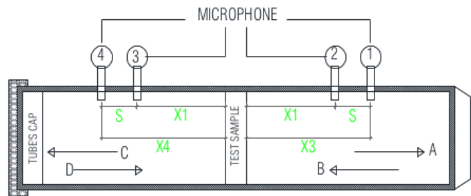
Gambar 3.3. Bagian Tabung Impedansi untuk Uji Kehilangan Transmisi Suara dengan empat mikrofon (17)
