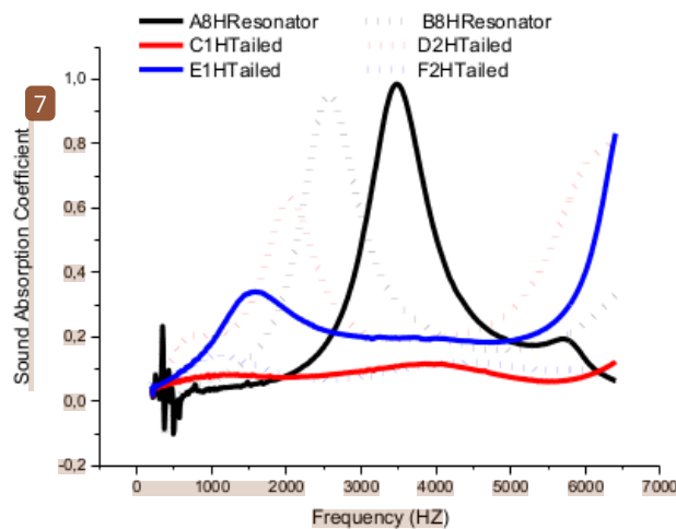
Gambar 4.7. Perbandingan absorpsi serat sabut kelapa dengan pajang gelombang resonator dan Hemp-Kenaf dengan rongga berekor[28]
