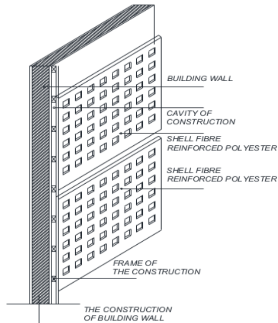
Gambar 3.17 Double skin construction design dengan material FRP cangkang kerang[13]
