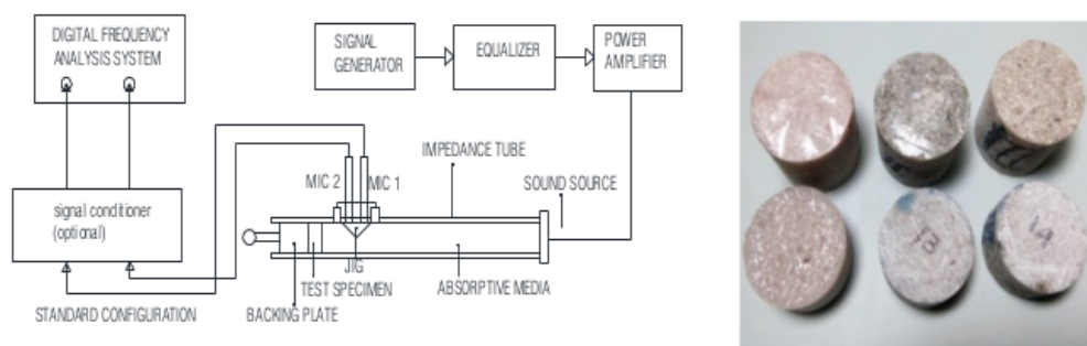
Gambar 3.2. (a) Konfigurasi uji tabung impedansi mengacu pada ASTM E 1050-98 [14] (b) Sampel uji Shell Fiber Reinforced Polyester (SFRP) [13]
