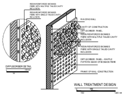
Gambar 4.13. Aplikasi serat hemp dan kenaf pada interior bangunan[28]
