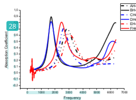
Gambar 3.5. Koefisien penyerapan cangkang komposit dengan 4 resonator[13]
