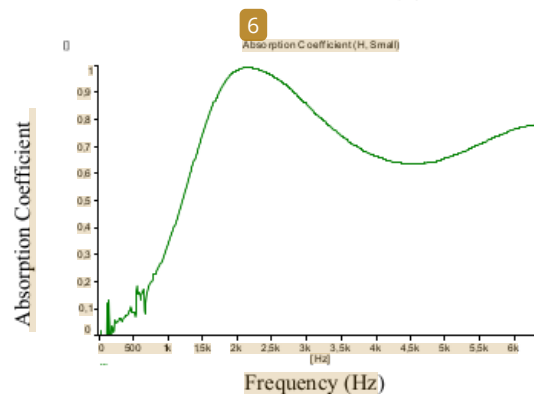
Gambar 5.2. Koefisien Absorpsi beton foamed dengan cangkang kerang ebagai agregat halus
