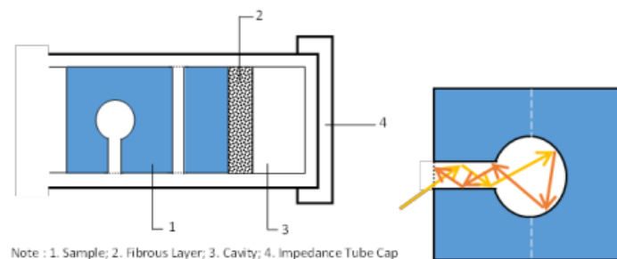
Gambar 4.5. Refleksi dan blok suara pada rongga[28]
