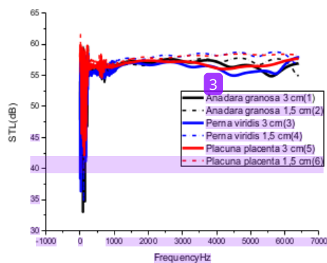
Gambar 3.9. STL SFRP tanpa perlakuan[13]
