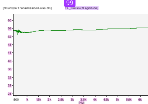
Gambar 2.5. Grafik STL mortar ringan cangkang kerang tebal 0.8 cm
