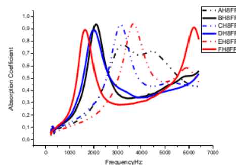
Gambar 3.7. Koefisien penyerapan cangkang komposit dengan FR (Fibrous Layers)[13]
