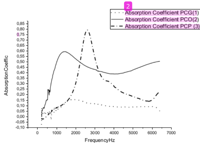
Gambar 2.13. Grafik Perbandingan Koefisien Absorpsi material
