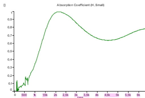
Gambar 2.4. Grafik Koefisien Absorpsi mortar cangkang kerang tebal 1.8 cm
