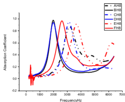
Gambar 3.6. Koefisien penyerapan cangkang komposit dengan 8 resonator[13]
