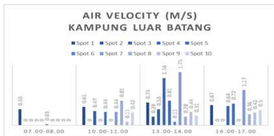
Fig. 5: Air Velocity in Kampung Luar Batang
