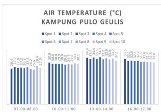
Fig. 6: Air Temperature in Kampung Pulo Geulis
