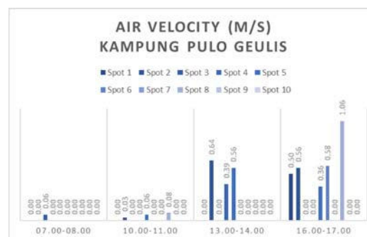
Fig. 8: Air Velocity in Kampung Pulo Geulis
