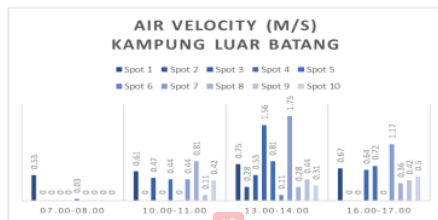
Fig. 5: Air Velocity in Kampung Luar Batang
