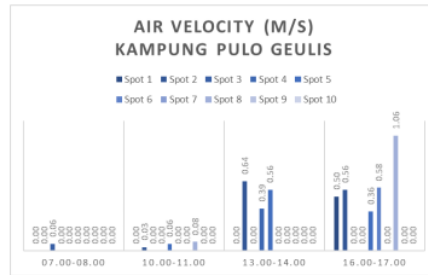
Fig. 8: Air Velocity in Kampung Pulo Geulis
