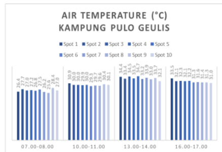
Fig. 6: Air Temperature in Kampung Pulo Geulis
