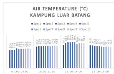
Fig. 3: Air Temperature in Kampung Luar Batang.
