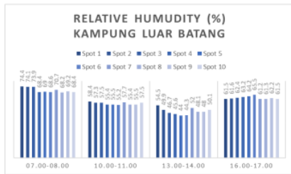
Fig. 4: Relative Humidity in Kampung Luar Batang
