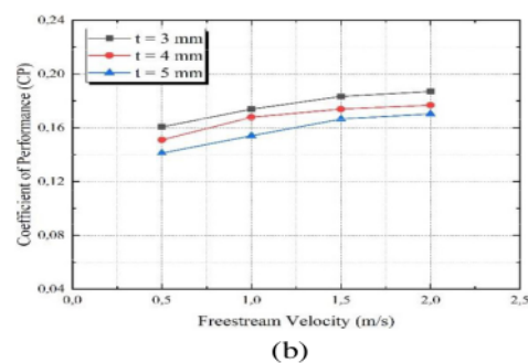
Gambar 8. Performa turbin sebagai fungsi kecepatan freestream untuk turbin Savonius konvensional (a) koefisien torsi; dan (b) koefisien daya
