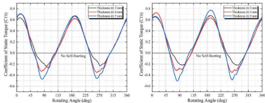
Gambar 10. Koefisien torsi statis C_{TS} sebagai fungsi sudut putar turbin untuk susunan turbin non-overlap dengan variasi tebal blade t = 3, 4 dan 5 \text{ mm}
