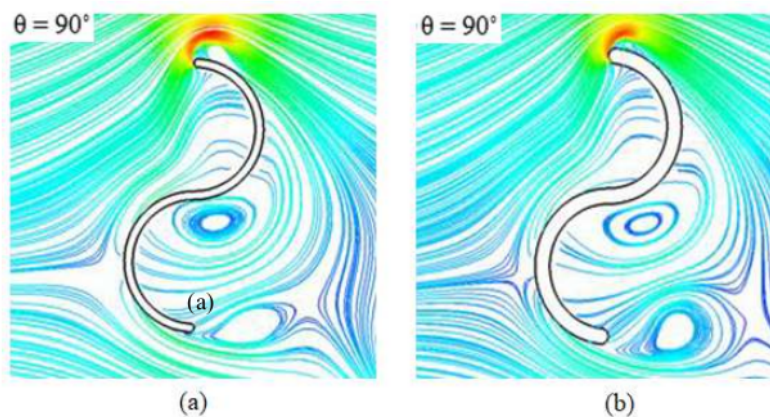
Gambar 5. Struktur aliran melewati turbin Savonius nonoverlap pada U_{\infty} = 0,5 m/s dengan sudut putar \theta = 90^\circ untuk (a) t = 3 mm; dan (b) t = 5 mm
