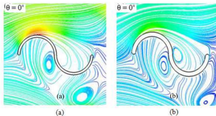
Gambar 4. Struktur aliran melewati turbin Savonius nonoverlap pada U_{\infty} = 0,5 m/s dengan sudut putar \theta = 0^\circ untuk (a) t = 3 mm; dan (b) t = 5 mm
