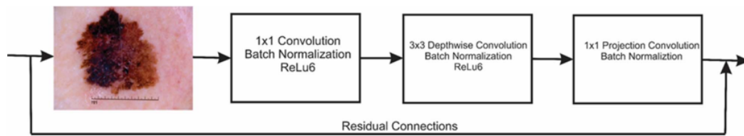
Fig. 3. Bottleneck layer of MobileNet v2
