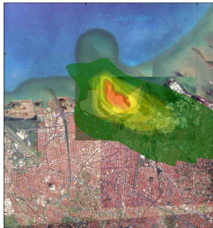
Gambar 5. Sebaran Emisi NOx dari Aktivitas Crane Pelabuhan Tanjung Mas
