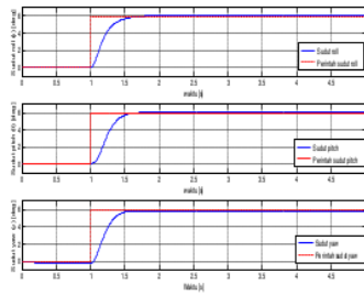
Gambar 18. Pengurangan masa 10% dan inersia 10%
