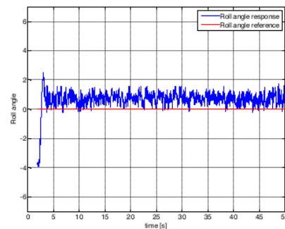
Gambar 21. Aplikasi HIL untuk respon roll dengan inisial kondisi 5^\circ
