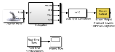
Gambar 13. Konfigurasi input joystick untuk aplikasi Pilot In the Loop (PIL)
