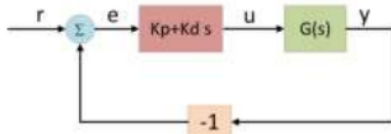
Gambar 2. PD kompensator
