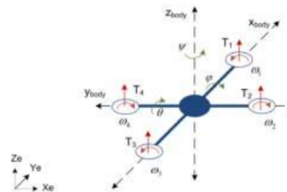
Gambar 1. Koordinat quadrotor
