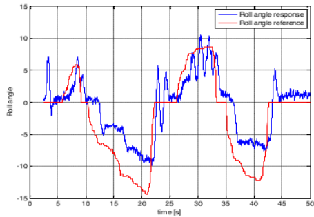
Gambar 22. Aplikasi PIL untuk respon roll
