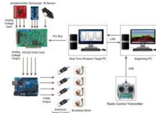
Gambar 7. Konfigurasi hardware HIL dan PIL
