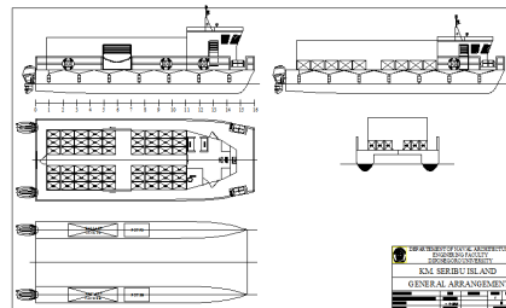
Gambar 3. Rencana Umum Kapal Pengangkut Ikan Katamaran
