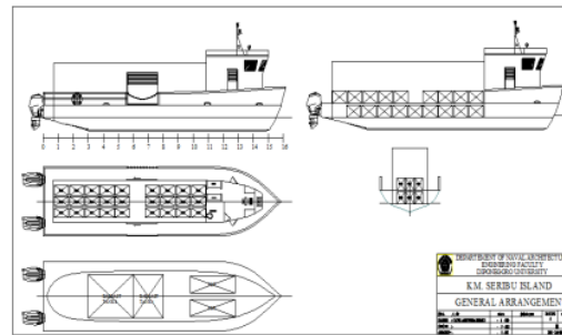
Gambar 2. Rencana Umum Kapal Pengangkut Ikan Monohull
