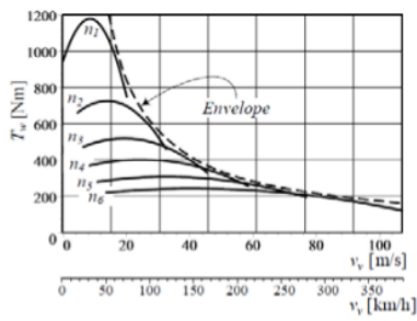
Gambar. 6. Plot torsi roda T_w sebagai fungsi kecepatan pada berbagai posisi transmisi.
