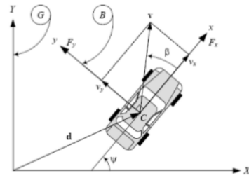
Gambar. 7. Kendaraan rigid pada bidang planar.
