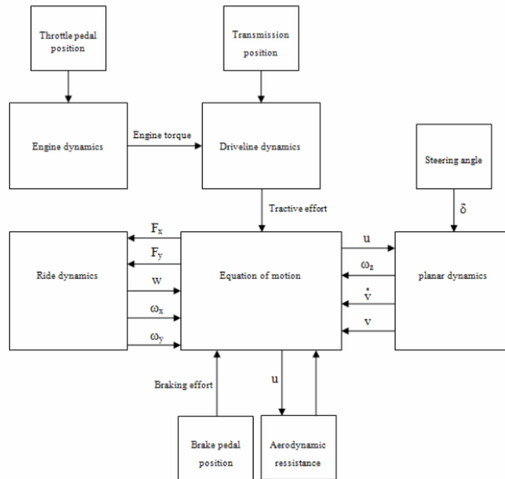
Gambar. 4. Skema interaksi berbagai model dinamik kendaraan bermotor.
