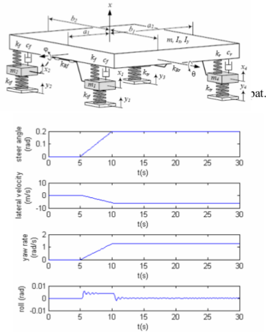
Gambar. 9. Plot skenario manuver dengan kecepatan konstan 30m/s.
