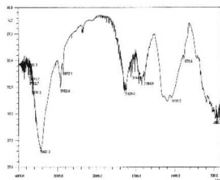
Gambar 7. senyawa hidrokarbon yang tersisa dalam proses pembakaran
