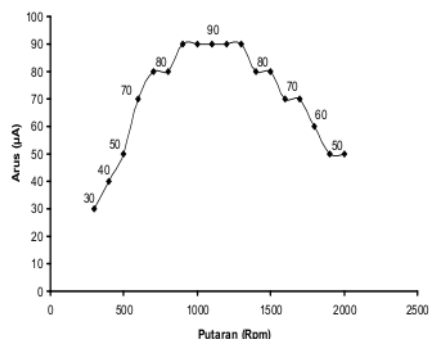
Gambar 2. Grafik Hubungan Antara Putaran Distributor Dan Arus
