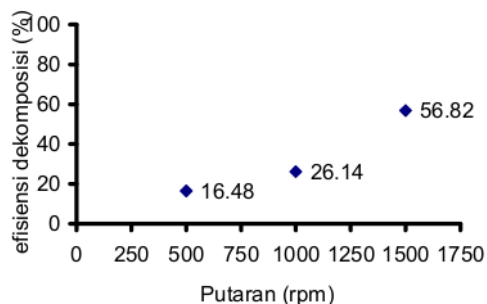
Gambar 5. Pengaruh putaran distributor terhadap efisiensi dekomposisi SO 2
