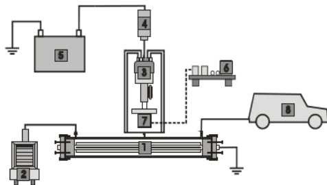
Gambar 1. Prototipe sistem pereduksi NO x dari gas emisi kendaraan bermotor. 1.Reaktor pembangkit plasma; 2. Gas Analyser; 3. Distributor; 4. Koil; 5. Aki; 6. Penyedia tegangan rendah DC; 7. Motor DC; 8. Kendaraan Bermotor
