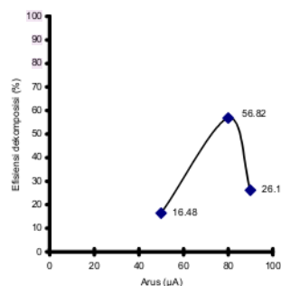
Gambar 6. Pengaruh arus terhadap efisiensi dekomposisi SO 2 .
